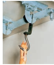
Rohrbahnen nach EU-Norm mit Sicherungsbügel für Eurohaken und Rohrbahnanschluß für direkte Verladung aus dem Schlachthaus.
